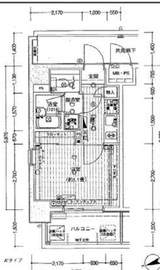
間取り
