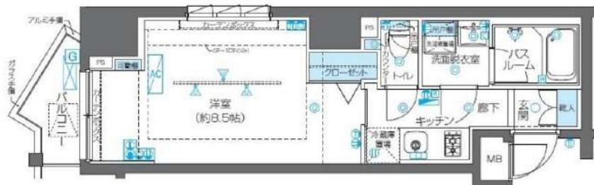
ZOOM渋谷笹塚/平面詳細図/A1・2・3・4タイプ
