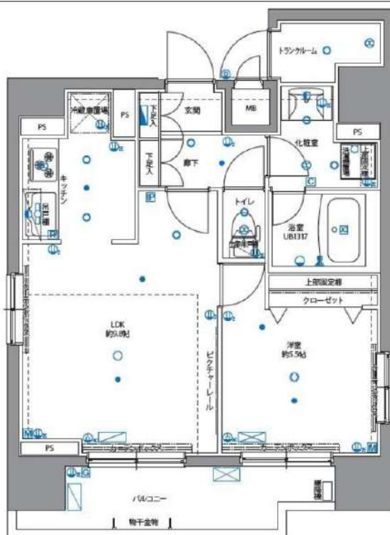
間取り図
